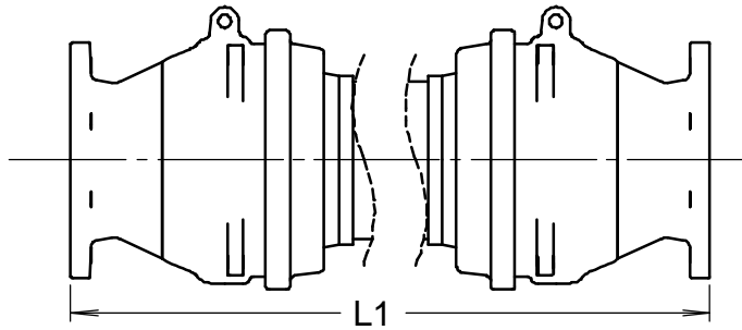
FLANGE X FLANGE
